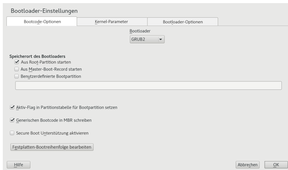
ABBILDUNG 11.5 CODE-OPTIONEN
