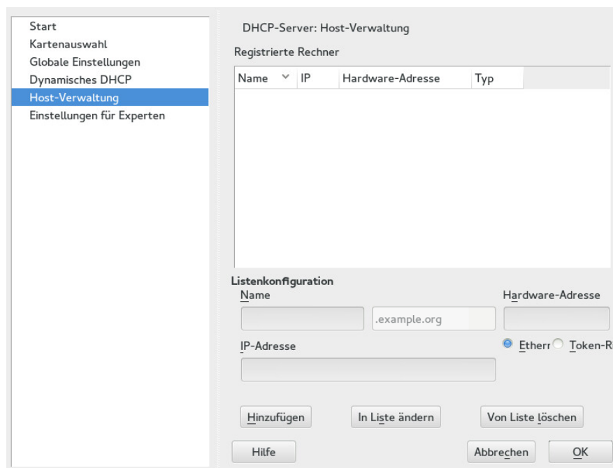
ABBILDUNG 24.5 DHCP-SERVER: HOST-VERWALTUNG
