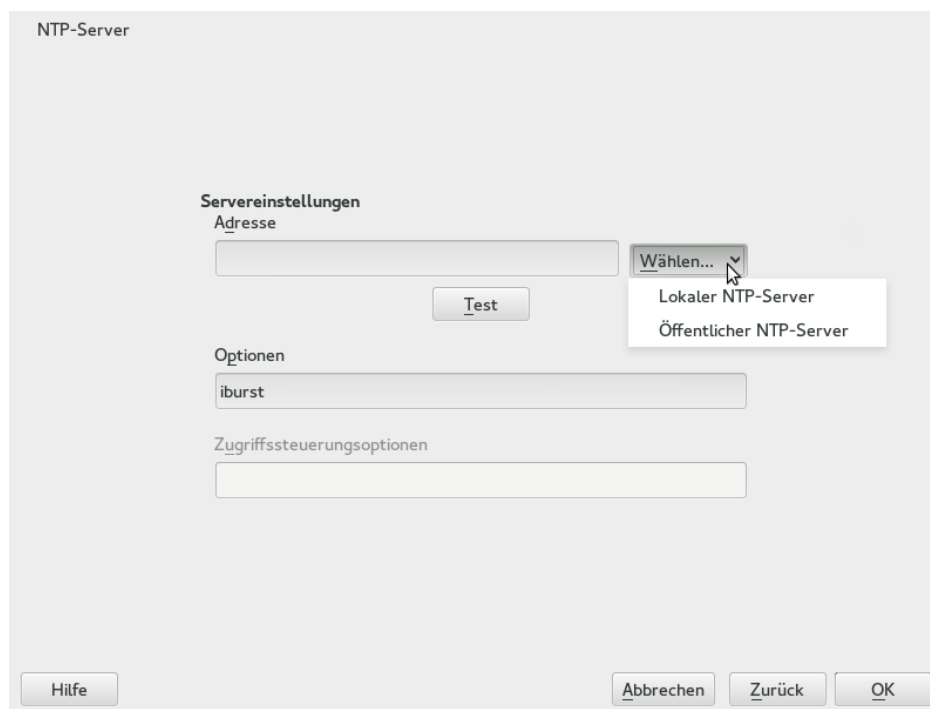
ABBILDUNG 22.1 YAST: NTP-SERVER
