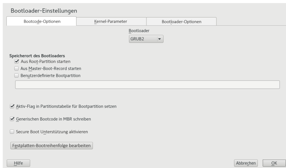
ABBILDUNG 11.2 BOOTCODE-OPTIONEN
