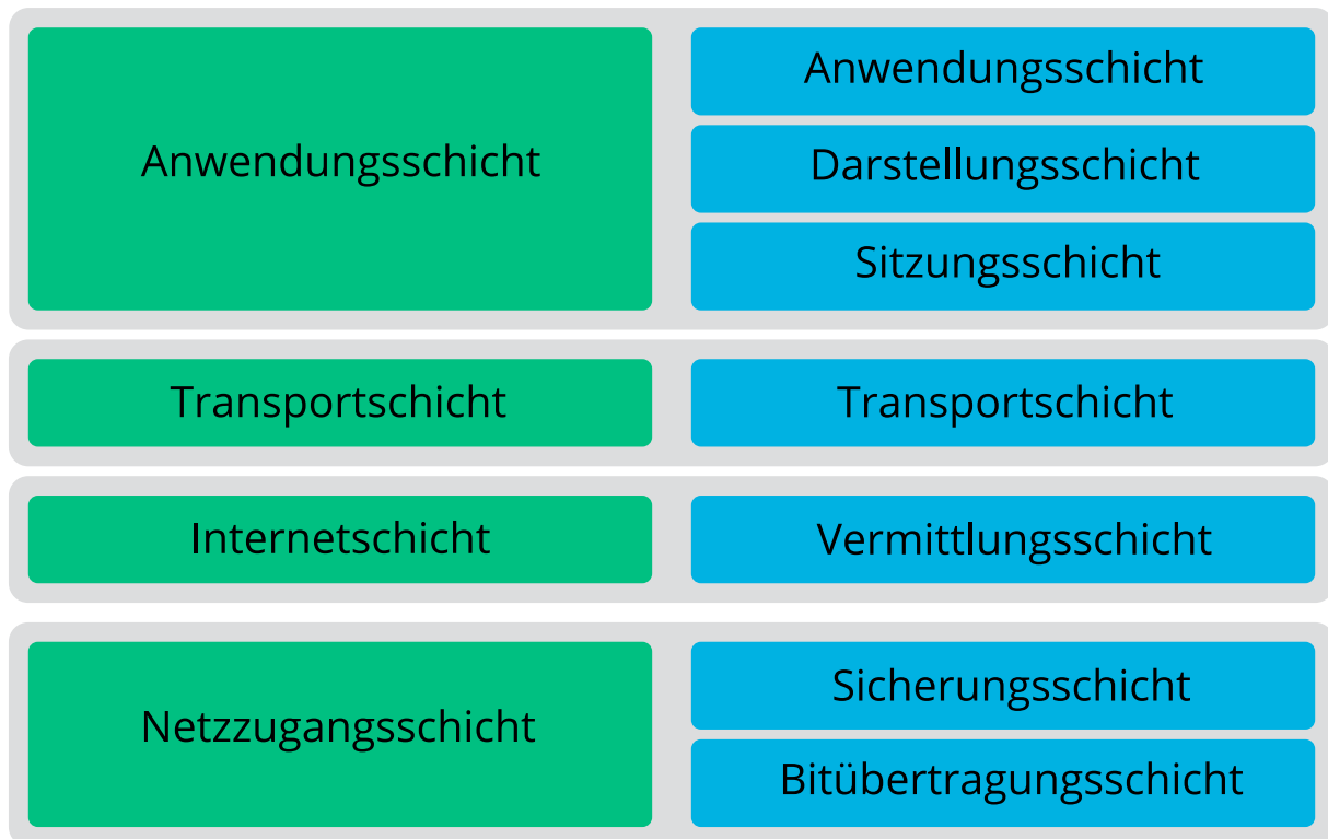
ABBILDUNG 15.1 VEREINFACHTES SCHICHTMODELL FÜR TCP/IP
