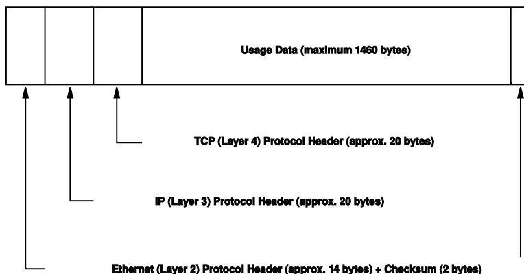
Figura 38.2 Pacote Ethernet TCP/IP
