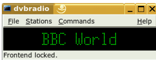
Figura 8.5 Rádio DVB
