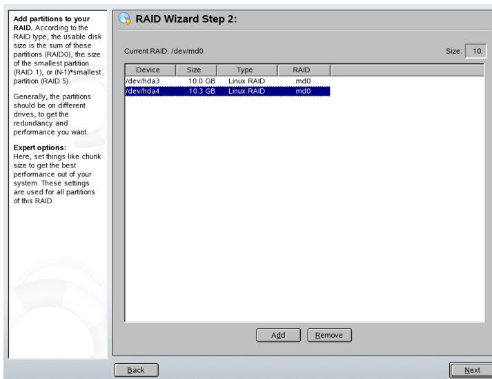
Figura 2.6 Partições RAID
