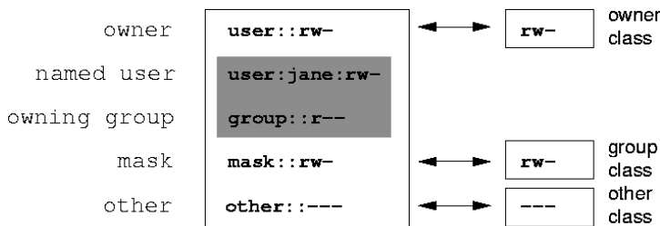
Figura 24.2 ACL estendida: entradas de ACL comparadas a bits de permissão
