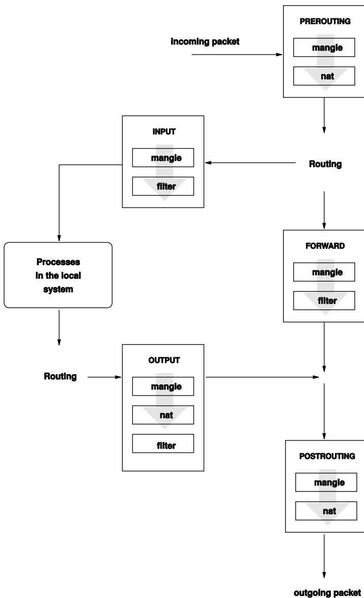
Figura 23.1 iptables: Caminhos possíveis de um pacote
