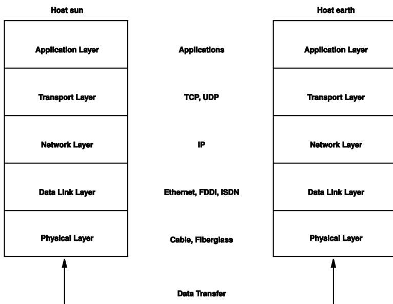
Figura 38.1 Modelo de camadas simplificado para TCP/IP
