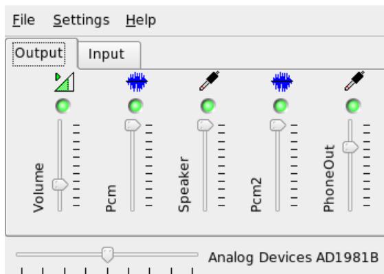
Figura 7.1 Mixer KMix
