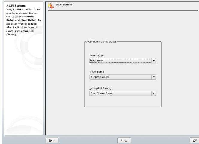
Figura 21.5 Configurações ACPI
